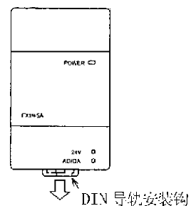
图 3.2: 直接安装
