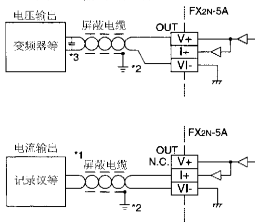
图 5.3: 输出的接线
