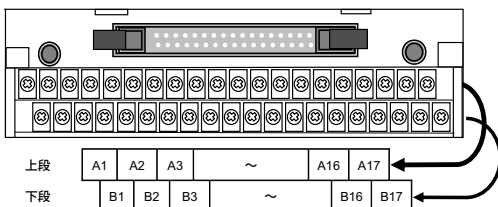
端子台変換ユニット 形 XW2D-34G6
