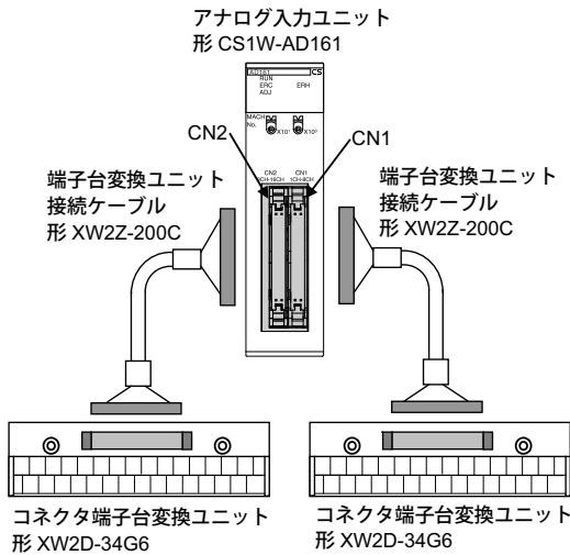
端子台変換ユニット 形 XW2D-34G6
